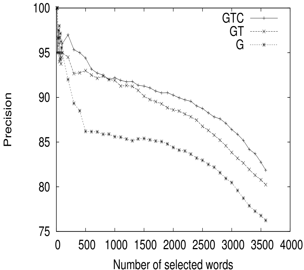
図2 14初期単語の場合の精度(%)。
