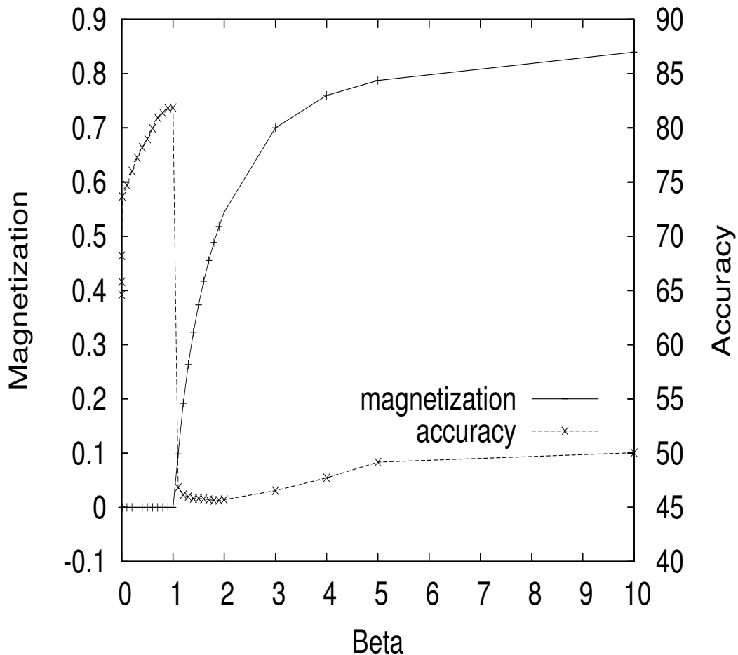
図1 平均磁化と正解率の変化 (14 初期単語).
