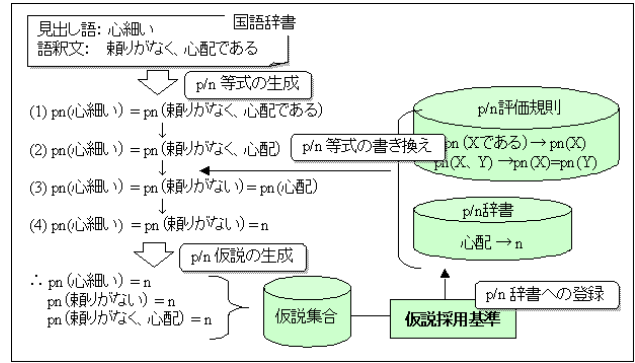
図 4: p/n 辞書獲得処理の流れ
